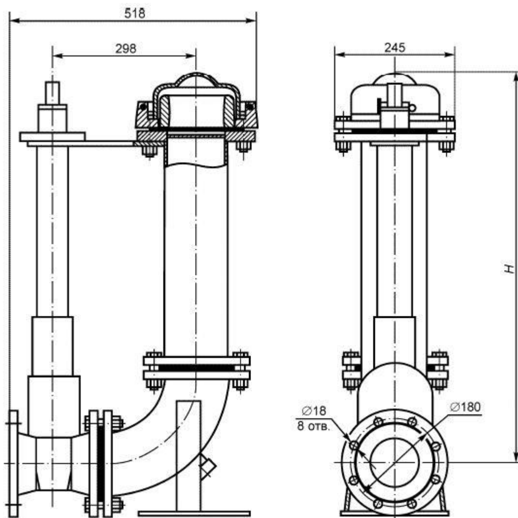
Рисунок А.2 - Гидрант пожарный подземный
